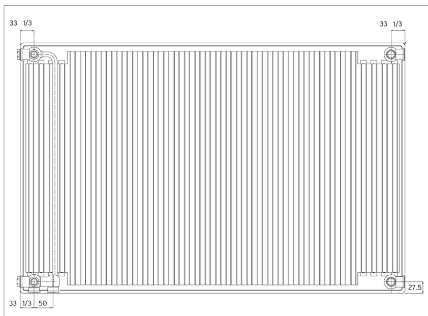
Tip radijatora 33
