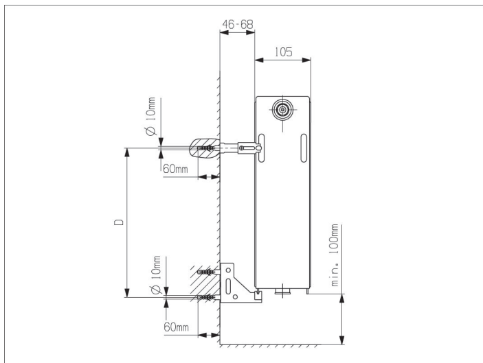
Tip radijatora 21, 22
