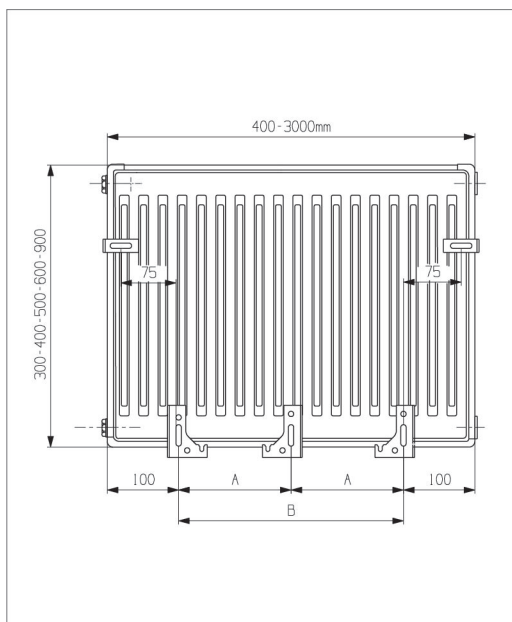
Tip radijatora 21, 22
